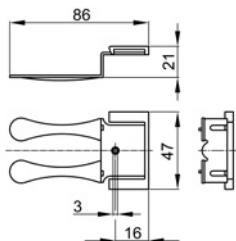
Easy-Clip, enkel anslutning till golvboxar
