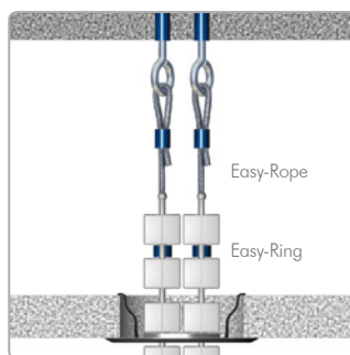
Montering av 2x KS Cube på innertak
