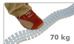
Tramsäker Tramphållfasthet utsträckt upp till 70 kg Tramphållfasthet hoptryckt upp till 90 kg
