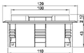
Easy-Outlet-TA för kablage
