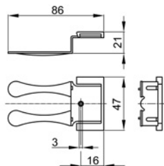
Easy-Clip, enkel anslutning till golvboxar
