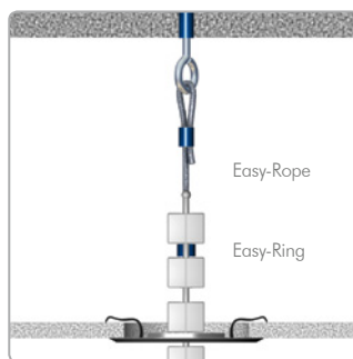
Montering med draglina på innertak
