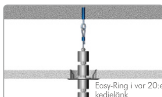
Innertaksupphängning med Easy-Rope och Easy-Ring
