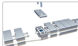
Easy-Stop-dragavlastning upp till 16 kablar
